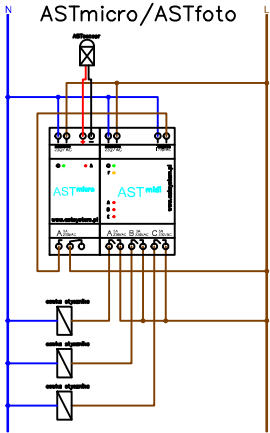
ASTmidi 3 wyjścia + ASTmicro/ASTfoto
