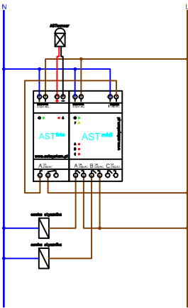
ASTmidi + ASTfoto
