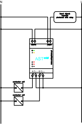
ASTmidi 2 outputs
