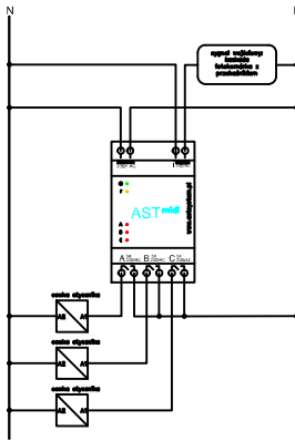
ASTmidi 3 wyjścia
