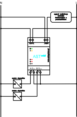
ASTmidi 2 wyjścia
